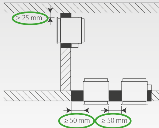
CCF rectangulaires (voir page 16)
