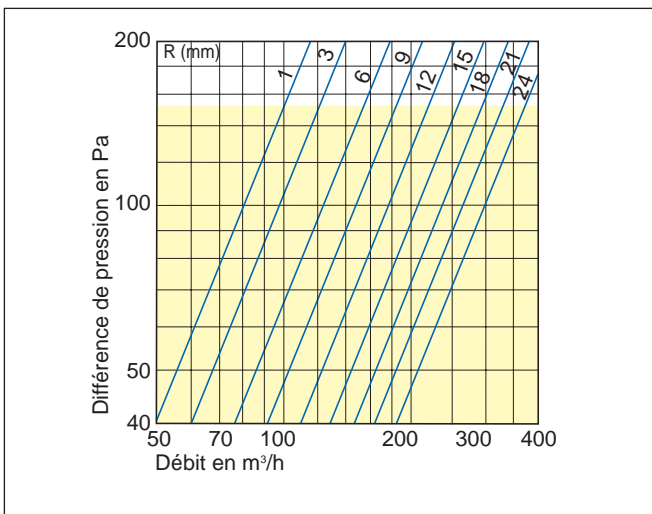
BIR 160
