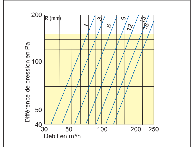
BIR 200
