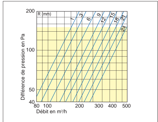
BIR 200
