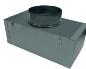
REBV Plénum de raccordement avec piquage axial
